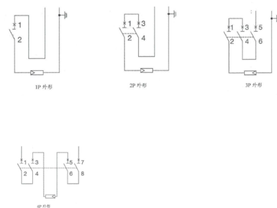
接线图:
